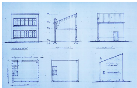
Bouwtekening van de zilversmidswerkplaats van de Gebr. van der Ree, later J. Gelderblom en Zn. Gemaakt door Aannemingsbedrijf Van der Pauw in 1977, kort voor de sloop, ten behoeve van een mogelijke wederopbouw op een andere plaats. Met dank aan Kees van der Pauw.
