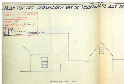
Detail uit de tekening van architect Died Visser voor het veranderen van de werkplaats van de heer P van Oostrom, goedgekeurd 7 mei 1947. Bestaande situatie aan de Havenstraat in 1947 van de 'nieuwere' werkplaats. Uiterst rechts de topgevel van de 'oude' werkplaats (NB) met 9-ruits venster.
