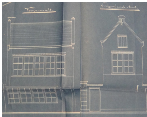
Varkensmarkt 4. Twee gevelaanzichten uit de tekening behorend bij de aanvraag Hinderwetvergunning van Driesen in 1905, voor de uitbreiding van zijn zilversmidswerkplaats met een verdieping.
